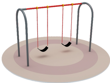
• Double Swing 305 x 106 x 213 cm
